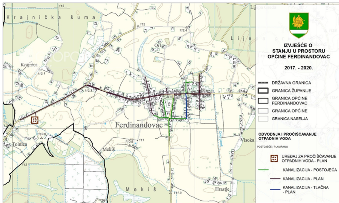
Slika 36. Sustav odvodnje i zbrinjavanja otpadnih voda
