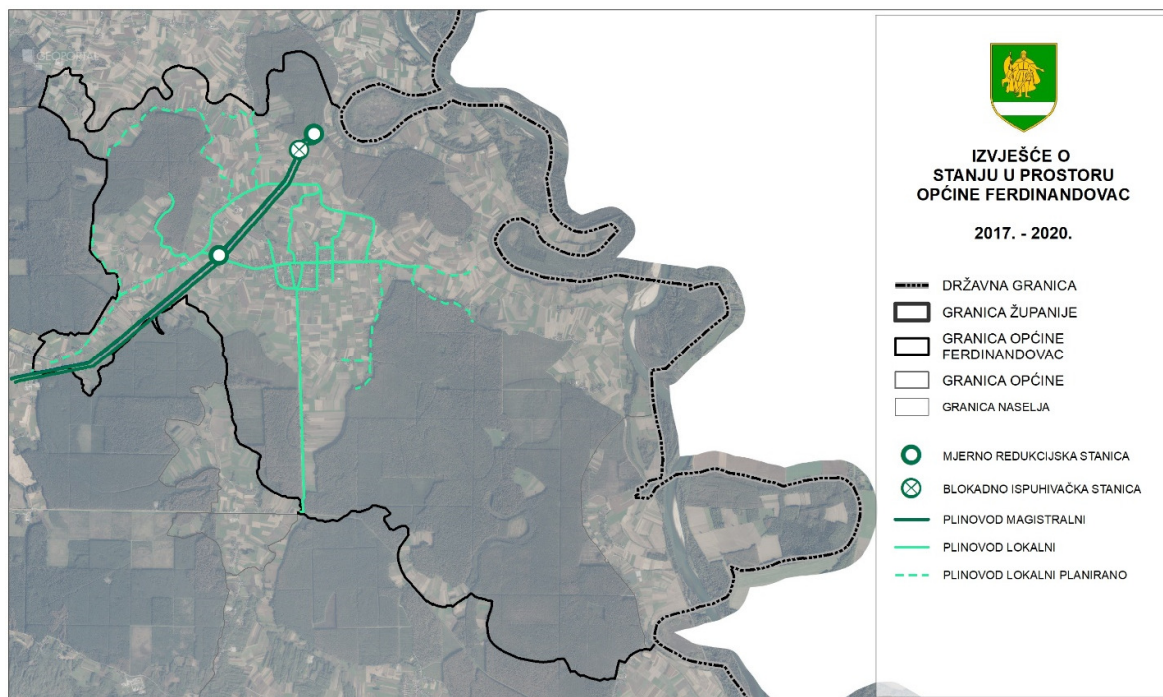
Slika 33. Plinovodi u sustavu tvrtke PLINACRO d.o.o te lokalna plinoopskrbna mreža
