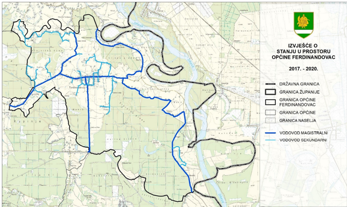
Slika 35. Javni vodoopskrbni sustav Općine Ferdinandovac
