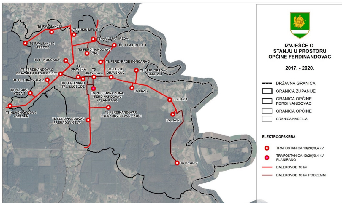
Slika 26. Elektroopskrbeni sustav na području Općine Ferdinandovac
