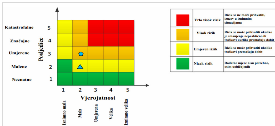
Slika 56. Matrica rizika - posljedice tehničko-tehnoloških nesreća
