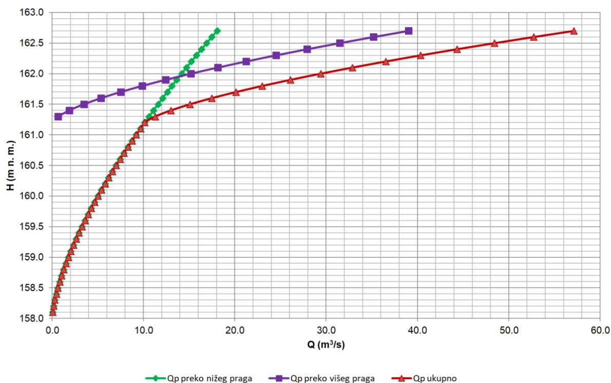
Grafički prikaz 3-21: Odnos protoka preko preljeva
