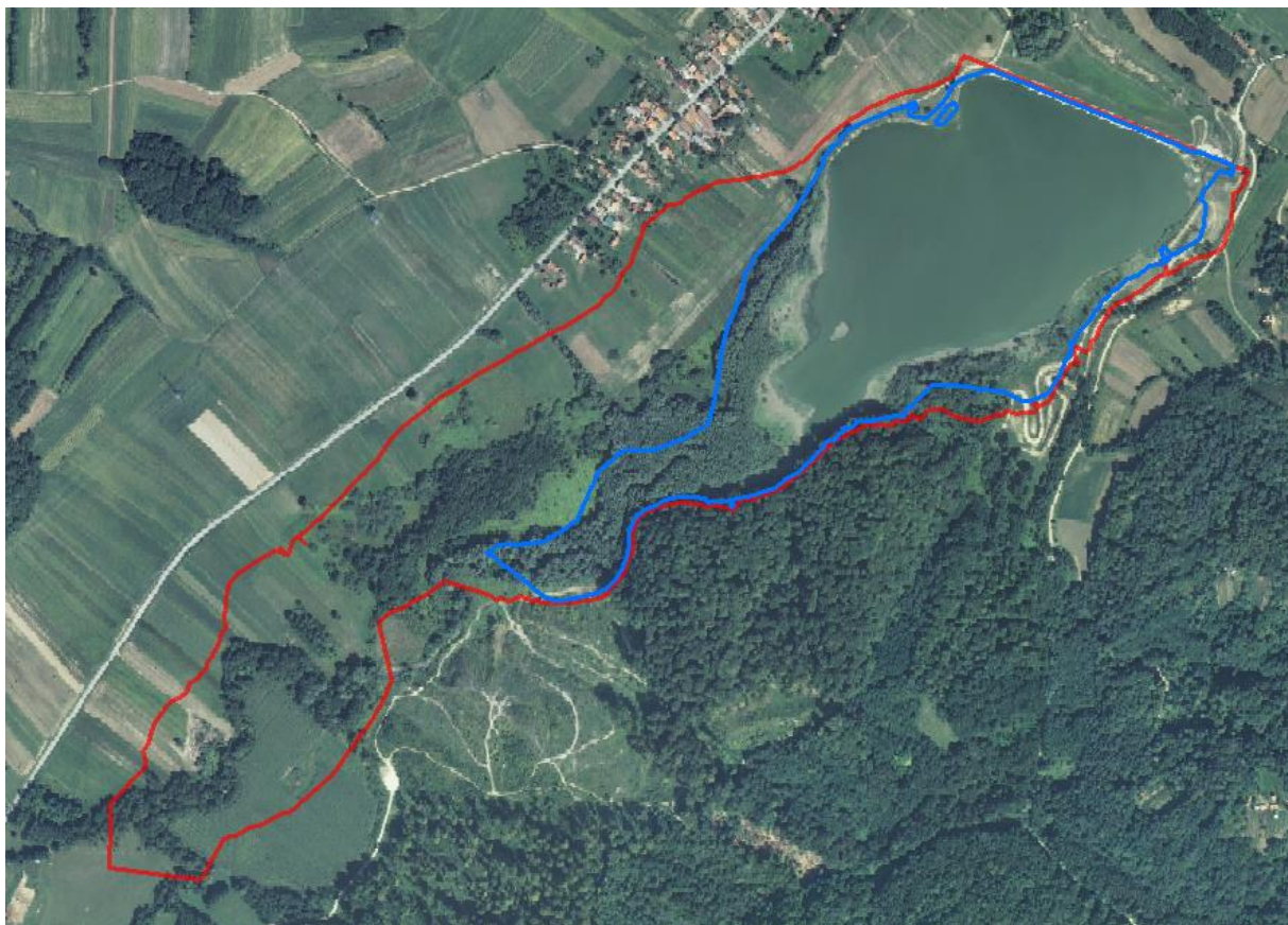
Grafički prikaz 3-22: Usporedba dosega vode za H=160.1 m n. m. (plava linija) i za H=162.7 m n. m. (crvena linija)
