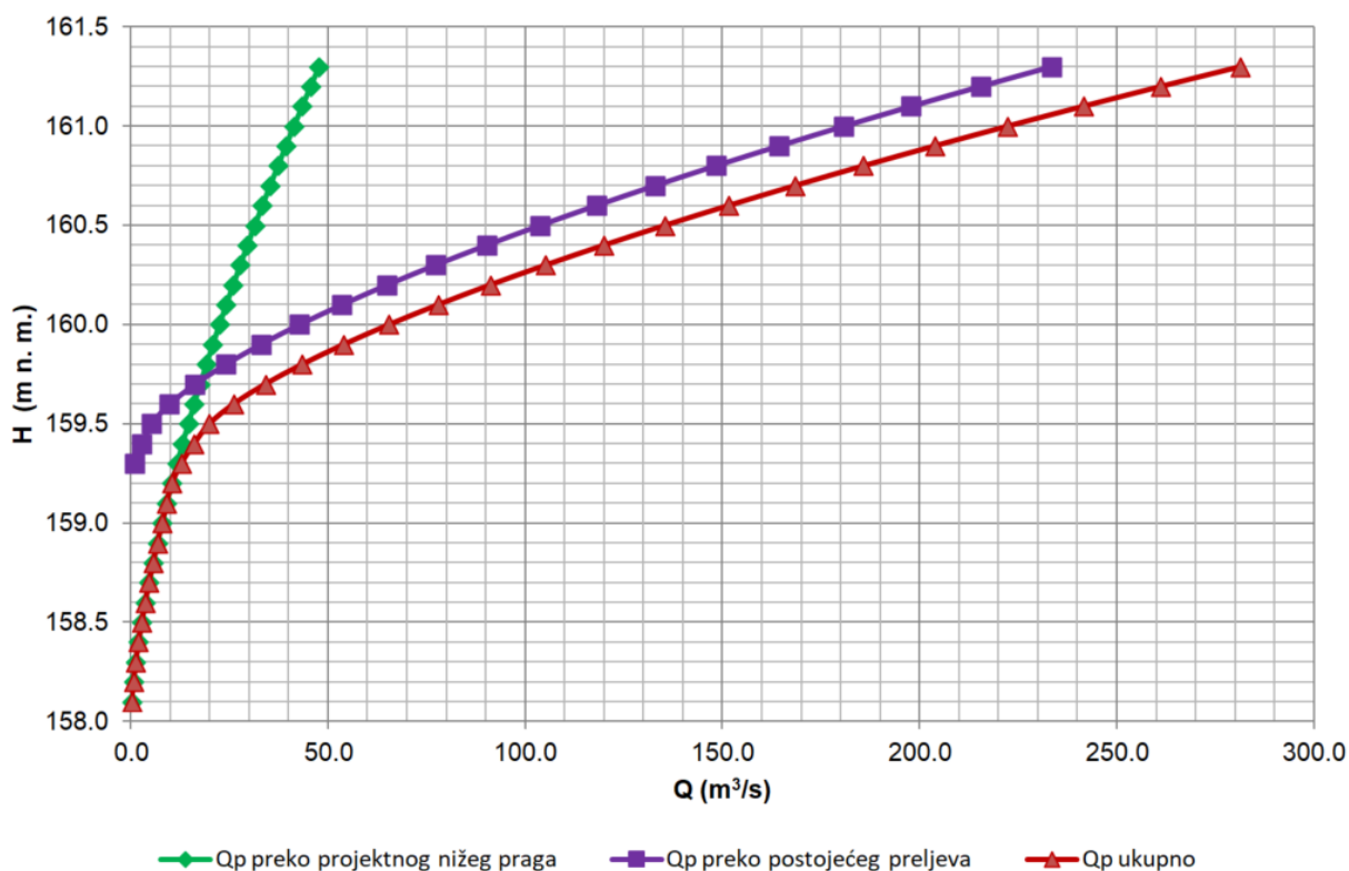
Grafički prikaz 3-19: Odnos protoka preko preljeva
