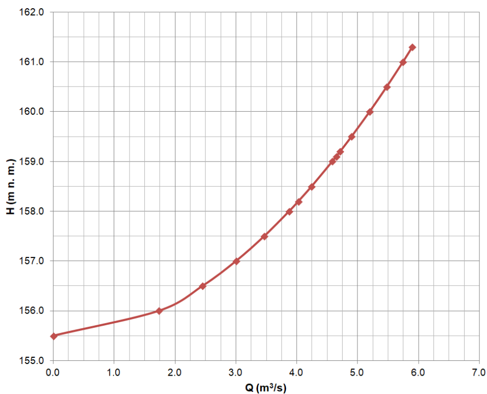
Grafički prikaz 3-14: Odnos razlike u visinama (H) i protoka kroz cijev (Q)
