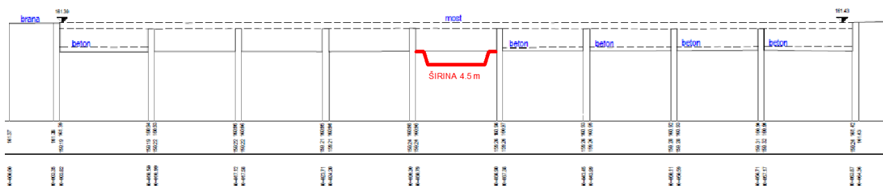
Grafčki prikaz 3-18: Uzdužni profil rekonstruiranog (stepenastog) preljeva
