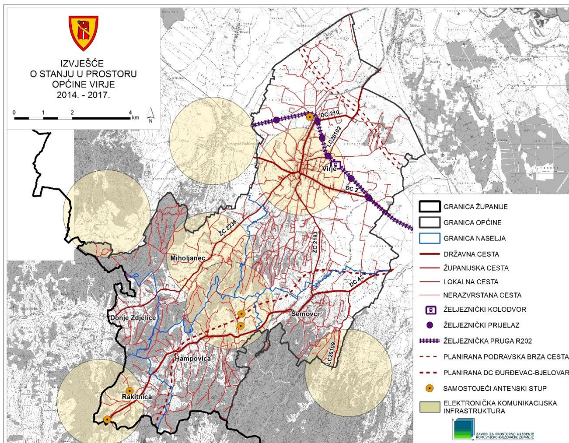
Slika 13 Infrastrukturni sustavi u Općini Virje
