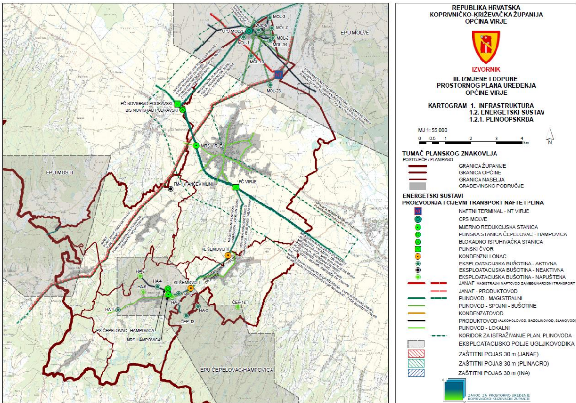
Slika 15 Kartogram „Energetski sustav – plinoopskrba“
