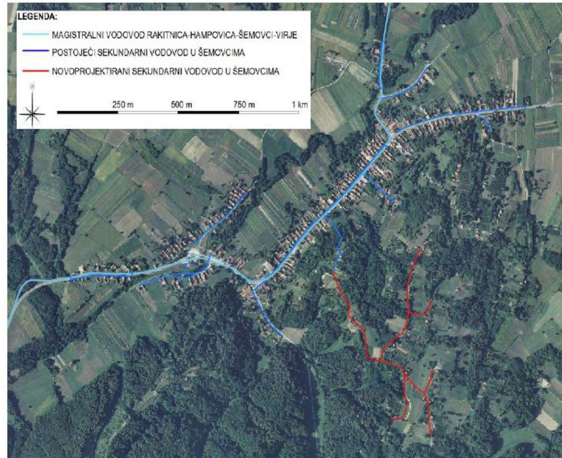
Slika 30 Prikaz planiranog zahvata izgradnje nove vodovodne mreže u naselju Šemovci
