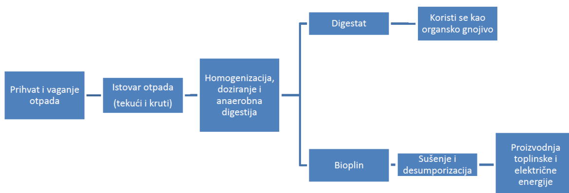
Slika 17 Shema tehnološkog procesa u bioplinskom postrojenju „Matvej“ d.o.o.
