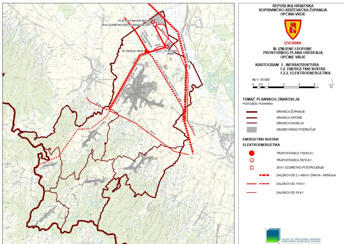
Slika 14 Kartogram „Energetski sustavi – elektroenergetika“
